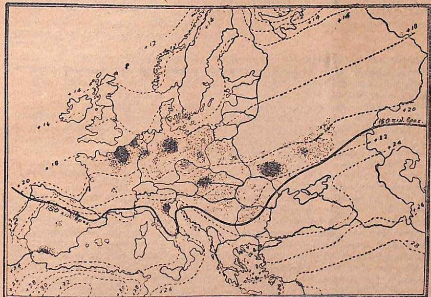
Εἰκ. 1.—Ἡ καλλιέργεια τοῦ ζαχαροτεύτλου ἐν Εὐρώπῃ (ἐκαστὴ στιγμή παριστᾷ 4.000 στρέμματα) αἱ ἰσοθερμοὶ τοῦ Ἰουλίου καὶ ἡ ἰσοπέτης τοῦ θέρους (Ἰούνιος, Ἰούλιος, Αὐγούστος) τῶν 150 χιλ. Κατὰ τὸν Harris (1)
