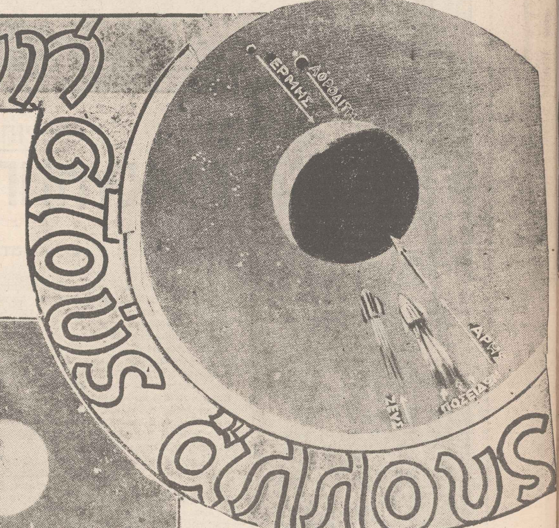
Αὐτὰ θὰ ἦτο ἡ κατεύθυνσις τὴν ὁποίαν θὰ εἶχαν αἱ ρουκέ- ται ἀπὸ τὴν Σελήνην πρὸς τὴν Γῆν
