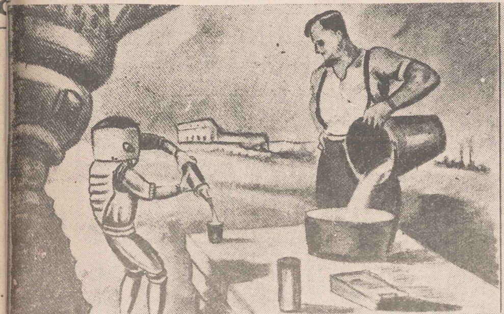
Ὁ κάτοικος τῆς Σελήνης, ἐάν ὑπῆρχε, θὰ ἦτο πολὺ μικρὸς καὶ ἀσθενέστατος. Με πολὺν κόπον θὰ κατώρθωνε νὰ κινήσῃ μίαν φιάλιν. Με τὴν ἰδίαν προσπάθειαν ἓνας κάτοικος τῆς Γῆς θὰ εἰμποροῦσε νὰ σπυρῇ ἓνα κουδάν γεμάτον νερὸ
