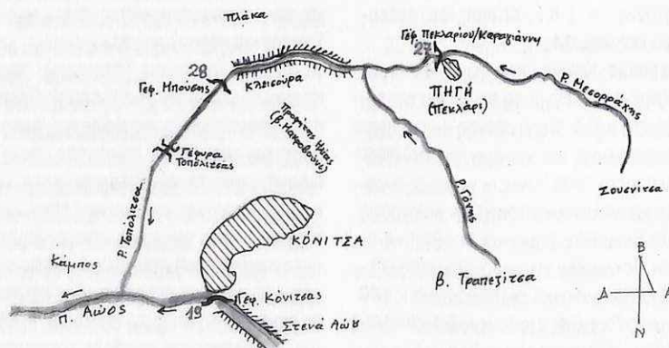
(ΠΣ-8) Το ποτάμιο σύστημα της περιοχής Πηγής - Κόνιτσας. [Πηγή: Ιχνογράφηση Θωμά Β. Ζιώγα, 2016]. "
