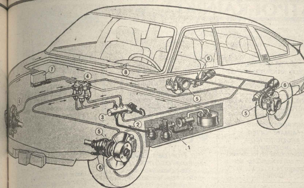
Μικροκομπιούτερ (με δίσκους) και σύστημα «αντιμπλόκ», που λειτουργεί με μικροκομπιούτερ (No 7)
