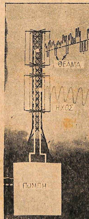
Πώς είναι κατασκευασμένη ή κεραία έκ- πομπής της τηλεόρασεως. Με την κεραία αυτή γίνεται συγχρόνως μεταδόσις ή- λεκτρομαγνητικών κυμάτων του ήχου και του θεάματος.
