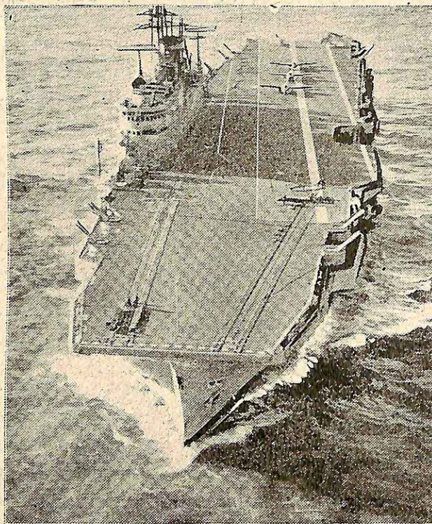
Μία αεροπορική φωτογραφία τοῦ πλέον συγχρονισμένου βρε- ταννικοῦ αεροπλανοφόρου «Βασιλικὴ κίβωτος», μετὰ τὸ γυνι- ῶδες κατὰστρωμά του, ποὺ διευκολύνει τὴν ὁμοδικὴν ἀπο- γείωσιν αεροπλάνων. Ἡ «Βασιλικὴ κίβωτος» δύναται νὰ φέρει δόμους ἀτομικὰς ἢ ὑδρογονικὰς καὶ περισσότερα τῶν πενήντα αεροπλάνων. Τὸ ἐκτόπισμά του εἶναι 36.800 τόνων.
