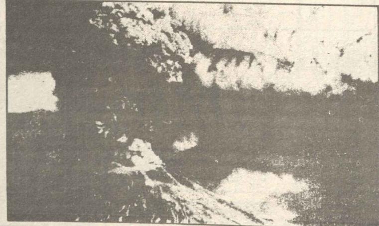
Κατά τις εκρήξεις των ηφαιστειών, απελευθερώνονται σημαντικές ποσότητες αεροζόλ, ουσίας που καταστρέφει το όζον.
