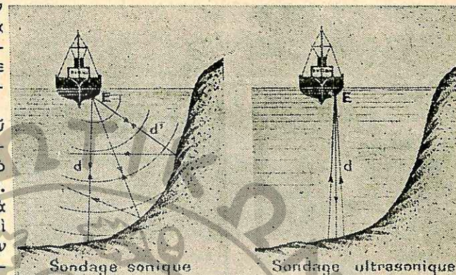
Σχηματική παράσταση ήχητικής βυθομέτρησης. Τα ήχητικά κύματα κτυπούν στο βυθό και επιστρέφουν στο πλοίο.
