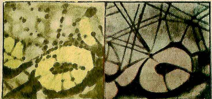
Τὰ περίφημα «κανάλια» τοῦ Ἄρεος κατὰ τὸν ἀστρονόμο Μαρτίνι δὲν εἶναι τίποτ' ἄλλο, παρὰ μιὰ ὀπτικὴ ἀπάτη...
