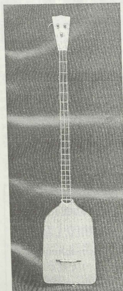
ΤΡΙΧΟΡΔΟΝ Ή ΠΑΝΔΟΥΡΙΣ Ηχείο: καρυδιά Καπάκι: έλατος Ντράτσο: σφενδάμι Ταστιέρα: έβενος Κεφαλή: κερασσιά Καβαλάρης: έβενος, κόκκαλο Χορδές: εβένινες Κλειδιά: έβενος Μήκος χορδής: 62 εκατ. Έτος κατασκευής: 1991
